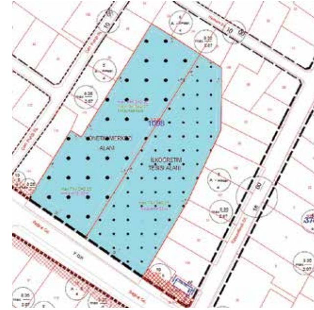
11.05.2006 onanlı 1/1000 ölçekli imar planı (1098 ada 2 parsel)
