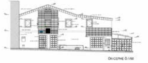
ÖN CEPHE 0:150
