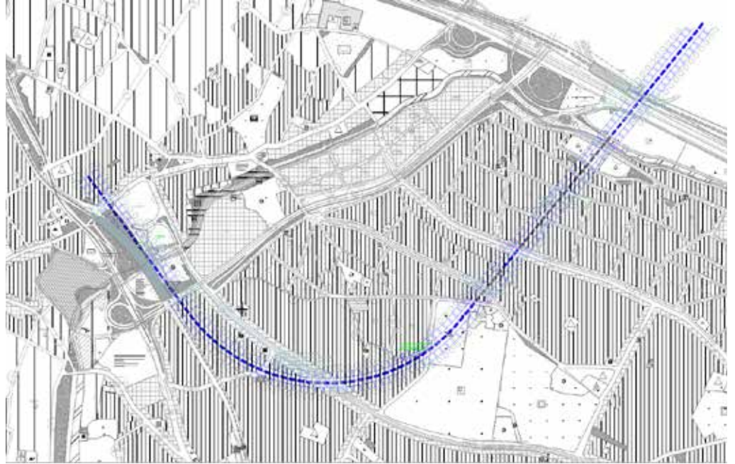
İstanbul, Metro ve Karayolu Boğaz Geçiş Projesi'ne ilişkin 1/5000 Ölçekli Nazım İmar Planı
